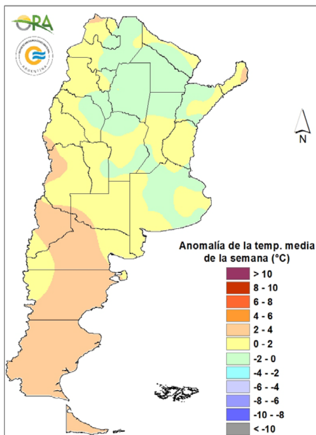
Anomalia de la temperatura media de la semana del 28/08/2024 al 03/09/2024
