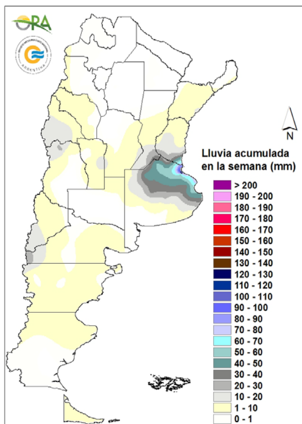
Precipitaciones acumuladas en la semana del 28/08/2024 al 03/09/2024
